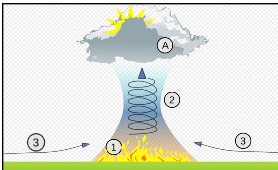
(1) fuoco, (2) convezione, (3) raffiche di vento, (A) piro-cumulonembo
